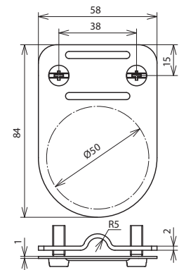
Maßbild TS 7.10 FL30 PP V2A
