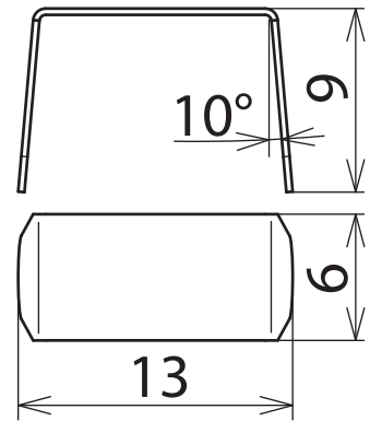
Maßbild NSE 8 V2A
