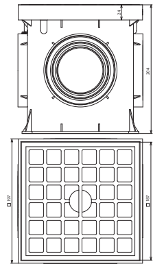
Maßbild UFTSK 197X197X204 K
