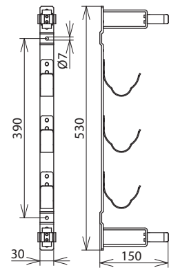
Maßbild HV 3HH SZ ET
