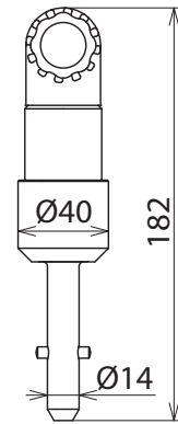
Maßbild AD SQ ZK 165
