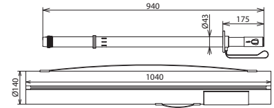
Maßbild HSA194 110 420 16.7
