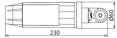
Maßbild ASP A 110 420 SL ZK
