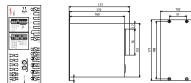
Maßbild DSRT DD CPS BACA
