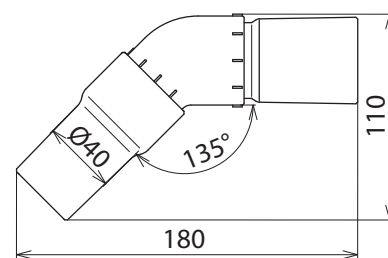
Maßbild SRW 135 MS
