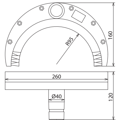
Maßbild HRB 190 MS
