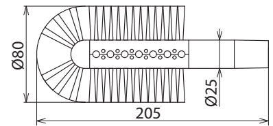
Maßbild STB 80 MS
