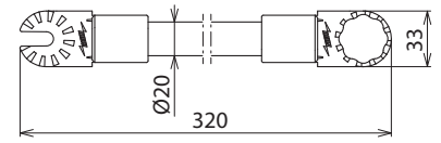
Maßbild ISV 320 ZK 123 SN7740
