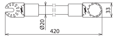
Maßbild ISV 420 ZK 123 SN7741
