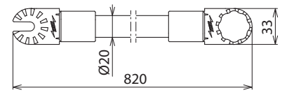
Maßbild ISV 820 ZK MS
