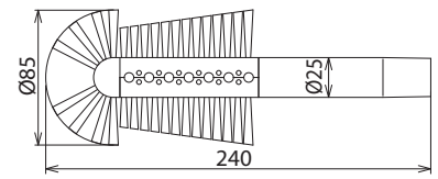
Maßbild STB 85 K NS
