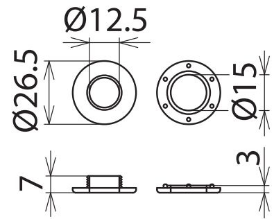
Maßbild OEK 12 NS
