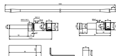
Maßbild HVI LI ASS RIV KF GFB1000 V2A
