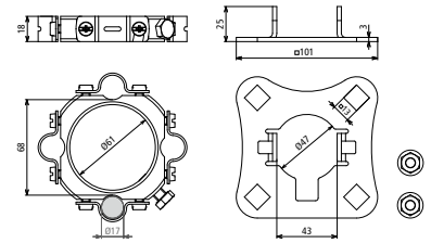
Maßbild BFS SR D50 4AE HVI LI AL V2A
