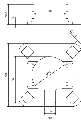
Maßbild AP SR D40 4AE HVI LI PL V2A
