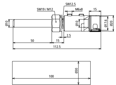
Maßbild AE BO10 KF HVI LI V2A
