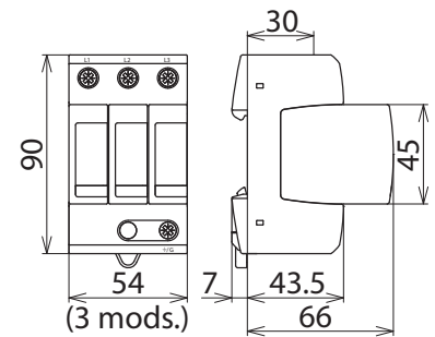
Maßbild DG MU 3PY 208 3W+G
