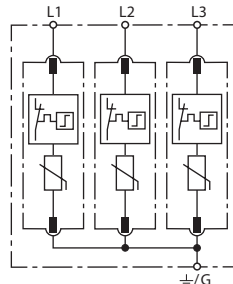
Prinzipialschaltbild DG MU 3PY 208 3W+G
