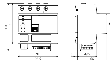
Maßbild DRC SD 2 1
