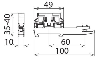
Maßbild SH1 18X3 ST
