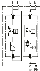
Prinzipschaltbild DG MD H TT 2P 275
