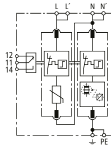
Prinzipschaltbild DG MD H TT 2P 275 FM
