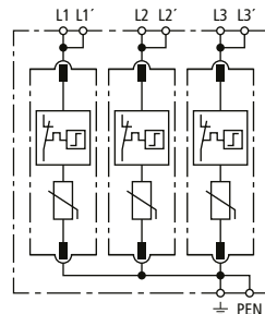
Prinzipschaltbild DG SMD TNC 275
