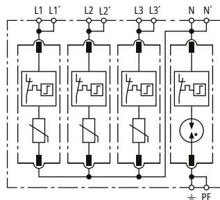
Prinzipschaltbild DG MD TT 275
