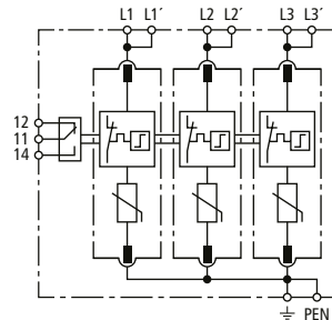
Prinzipialschaltbild DG MD TNC 150 FM
