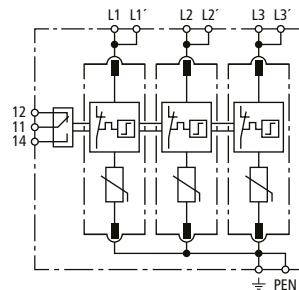
Prinzipschaltbild DG MD TNC 385 FM
