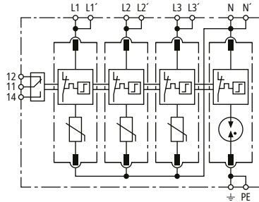
Prinzipialschaltbild DG MD TT 320 FM
