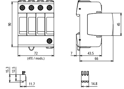
Maßbild DG MD TT 320 FM
