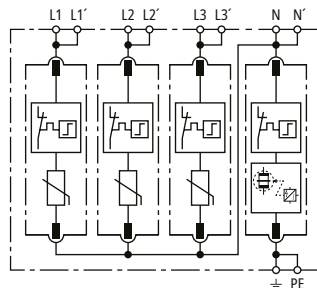
Prinzipschaltbild DG MD H TT 275
