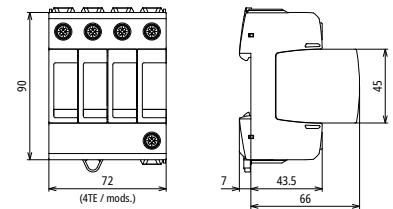
Maßbild DG MD H TT 275
