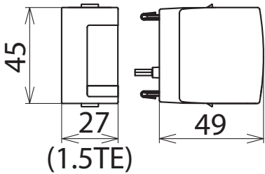
Maßbild DG MOD E DC 900
