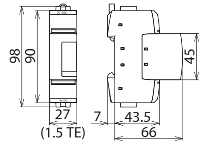
Maßbild DG SE DC 900
