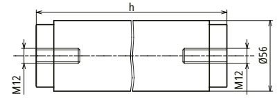
Maßbild SBKW 3/DH-I-0
