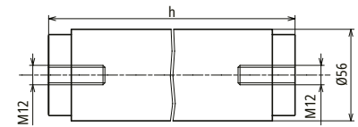
Maßbild SBKW 30/DH-I-0
