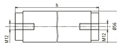
Maßbild SBKW 42/DH-I-0
