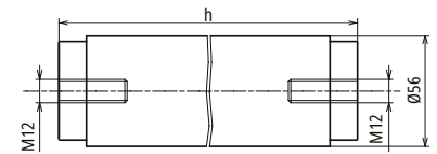
Maßbild SBKW 51/DH-I-0
