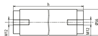
Maßbild SBKW 60/DH-I-0
