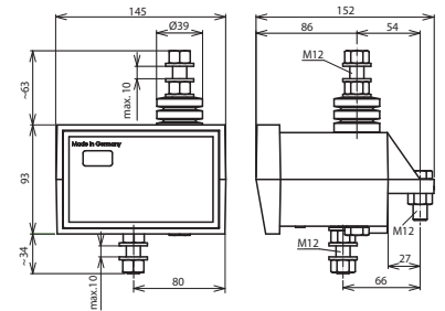
Maßbild DCC/RC 2
