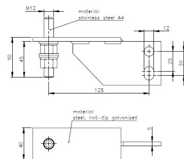
Maßbild SBKW AB15
