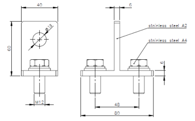
Maßbild SBKW-B PH2
