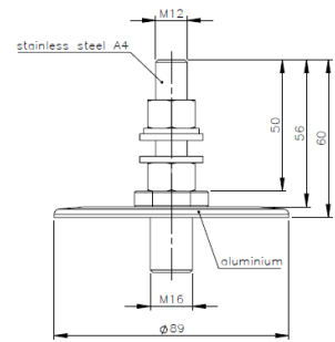
Maßbild SBKW-B PH4
