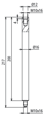
Maßbild
