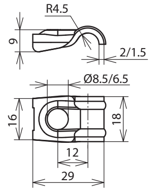
Maßbild
