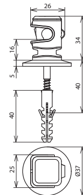
Maßbild
