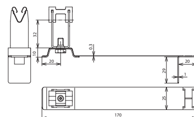
Maßbild
