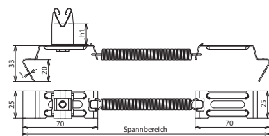
Maßbild
