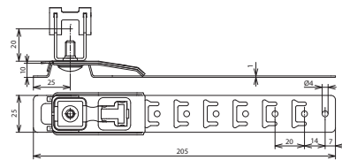
Maßbild
