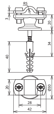
Maßbild
