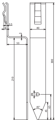
Maßbild
